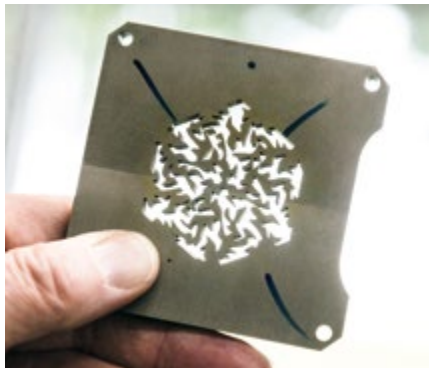
Präzisionsarbeit: Die exakte Kontur wurde mit einer Draherodiermaschine gefertigt.
