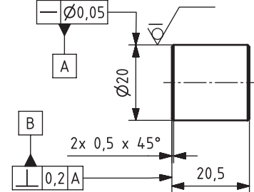
Skizze 6 \sqrt{Rz\ 16} \left(\sqrt{\quad}\right)
