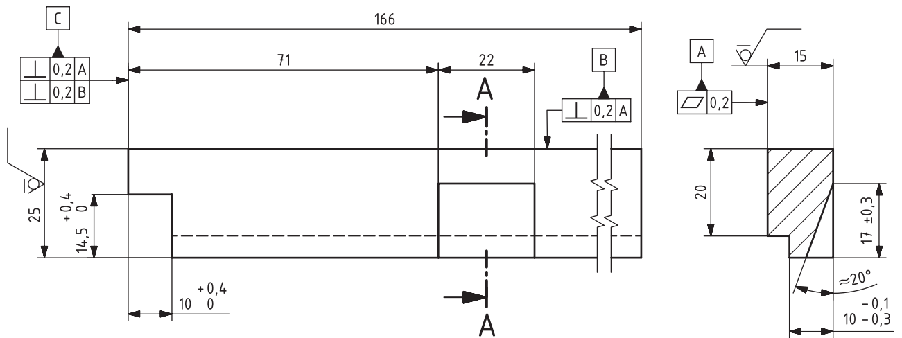
Skizze 2 \sqrt{Rz\ 16} \left(\sqrt{\quad}\right)
