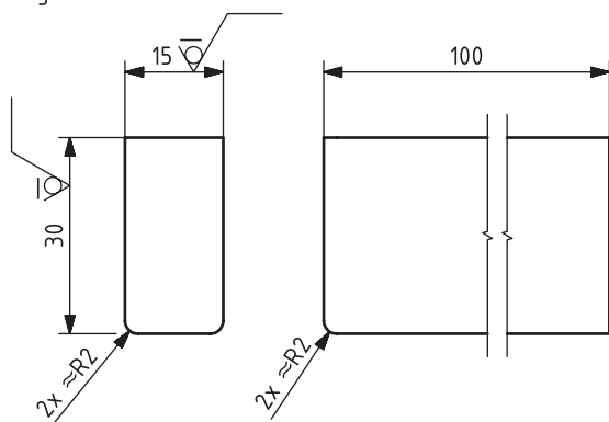
Skizze 9 \sqrt{Rz\ 16} \left(\sqrt{\quad}\right)
