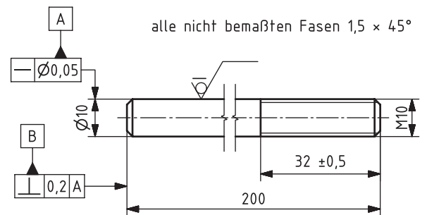
Skizze 6 \sqrt{Rz\ 16} \left(\sqrt{\quad}\right)
