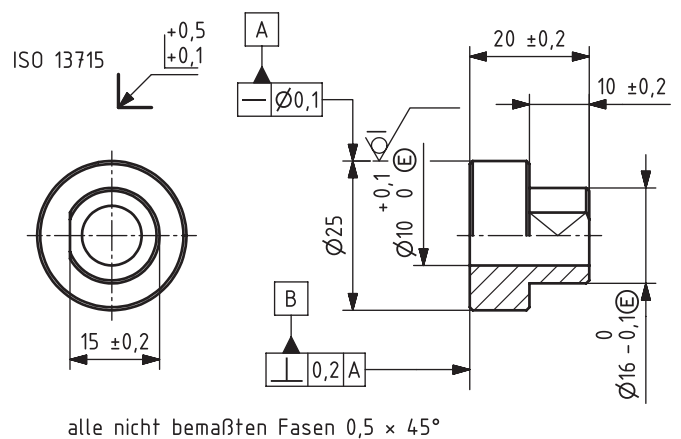
Skizze 7 \sqrt{Rz\ 16} \left(\sqrt{\quad}\right)
