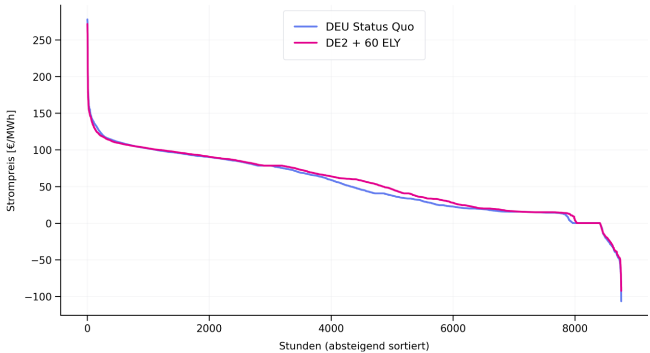
DEU Status Quo vs. DE2 + 60 ELY - Unterschiede sichtbar gemacht Gesamte Preisdauerlinie
