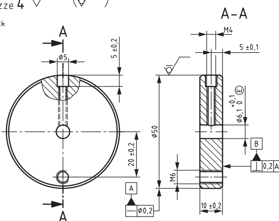
Skizze 4 \sqrt{Rz\ 25} ( \sqrt{\quad} )
