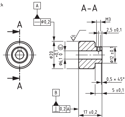
Skizze 2 \sqrt{Rz\ 25} ( \sqrt{\quad} ) alle nicht bemaßten Fasen 1 \times 45^\circ
