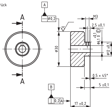
Skizze 5 \sqrt{Rz\ 25} ( \sqrt{\quad} )
