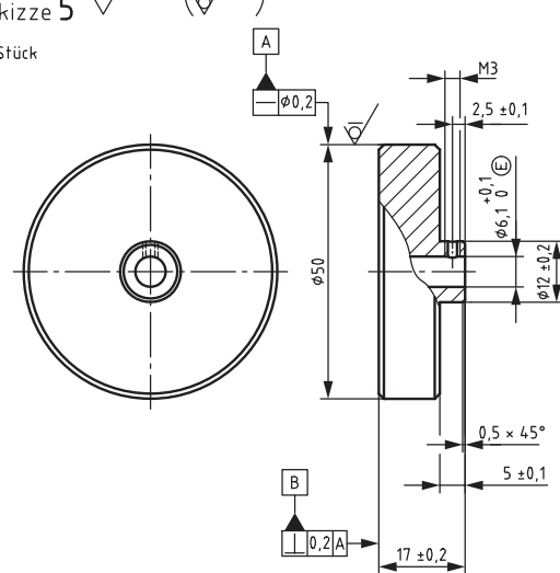
Skizze 5 \sqrt{Rz\ 25} ( \sqrt{\quad} )
