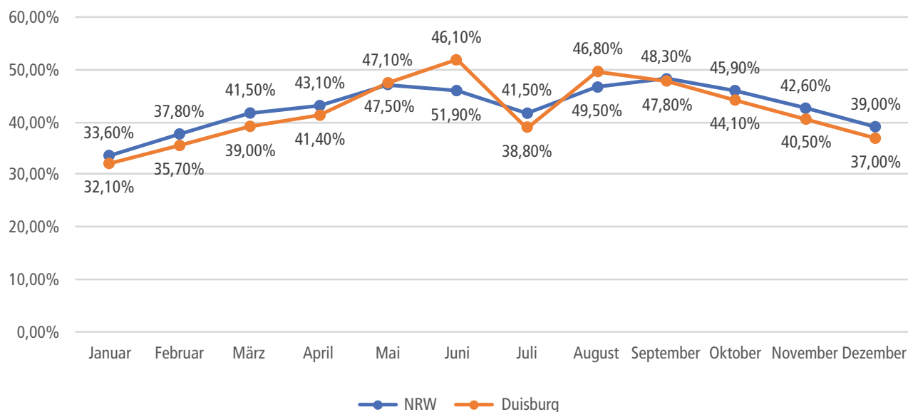
Abbildung 19: Auslastungsgrad in Duisburg und NRW 2023 19
