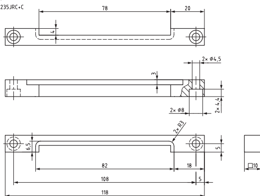
Leiste 1 2 Stück, S235JRC+C
