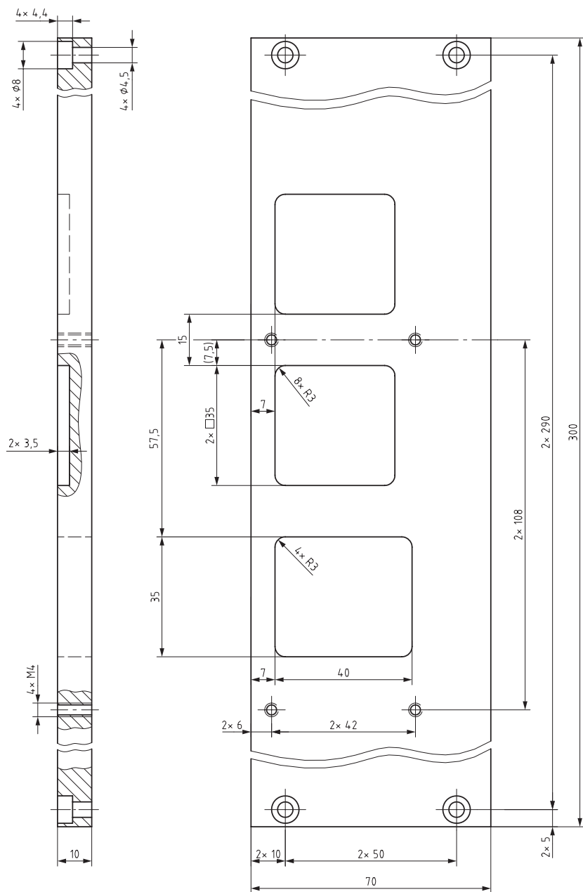
Leiste 1 2 Stück, S235JRC+C
