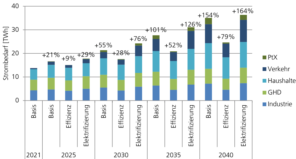
Abbildung 1: Projizierter Strombedarf von 2021 bis 2040 in Strombedarf der Region Stuttgart für die drei Szenarien Basis, Effizienz und Elektrifizierung
