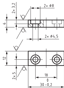
Skizze 3 \sqrt{Rz\ 16} (V) 2 Stück
