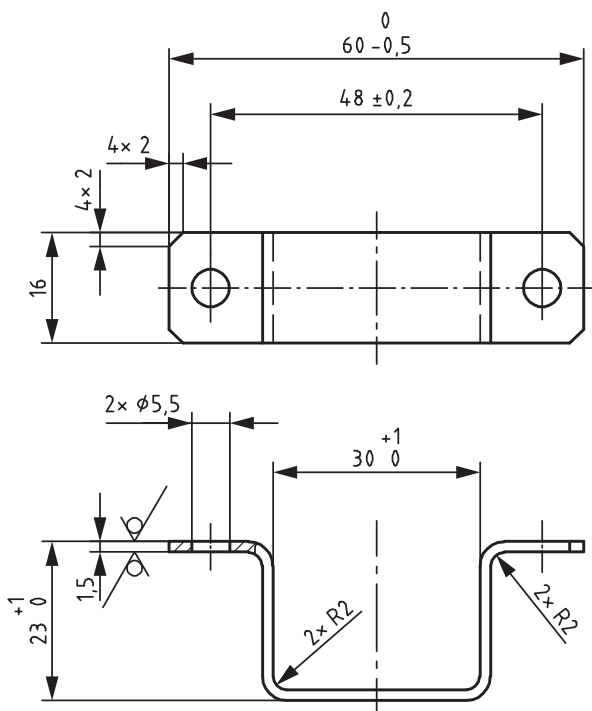
Skizze 3 \sqrt{Rz\ 16} ( \checkmark )
