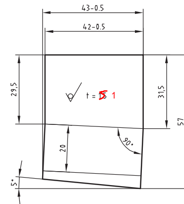
Skizze 8 \sqrt{Rz\ 16} (✓) 25.10.2023
