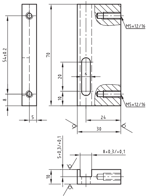
Skizze 4 \sqrt{Rz\ 16} (✓)
