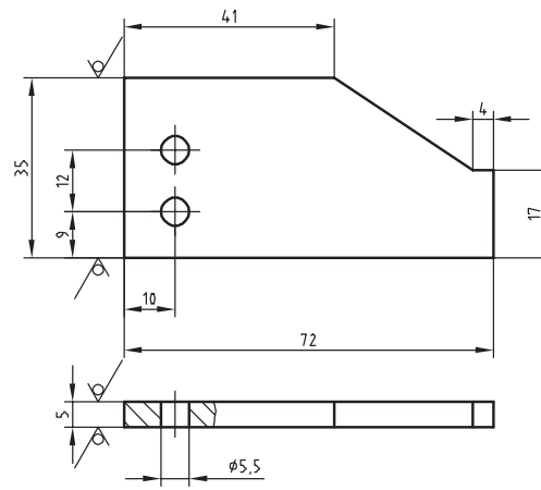
Skizze 5 \sqrt{Rz\ 16} (✓)
