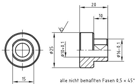
Skizze 9 \sqrt{Rz\ 16} (✓)
