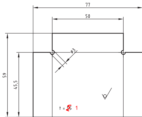
Skizze 7 \sqrt{Rz\ 16} (✓) 25.10.2023
