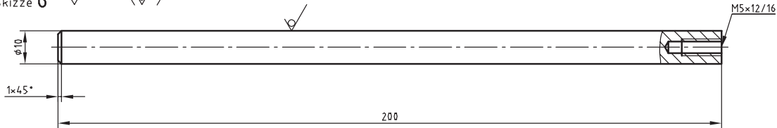
Skizze 6 \sqrt{Rz\ 16} (✓)
