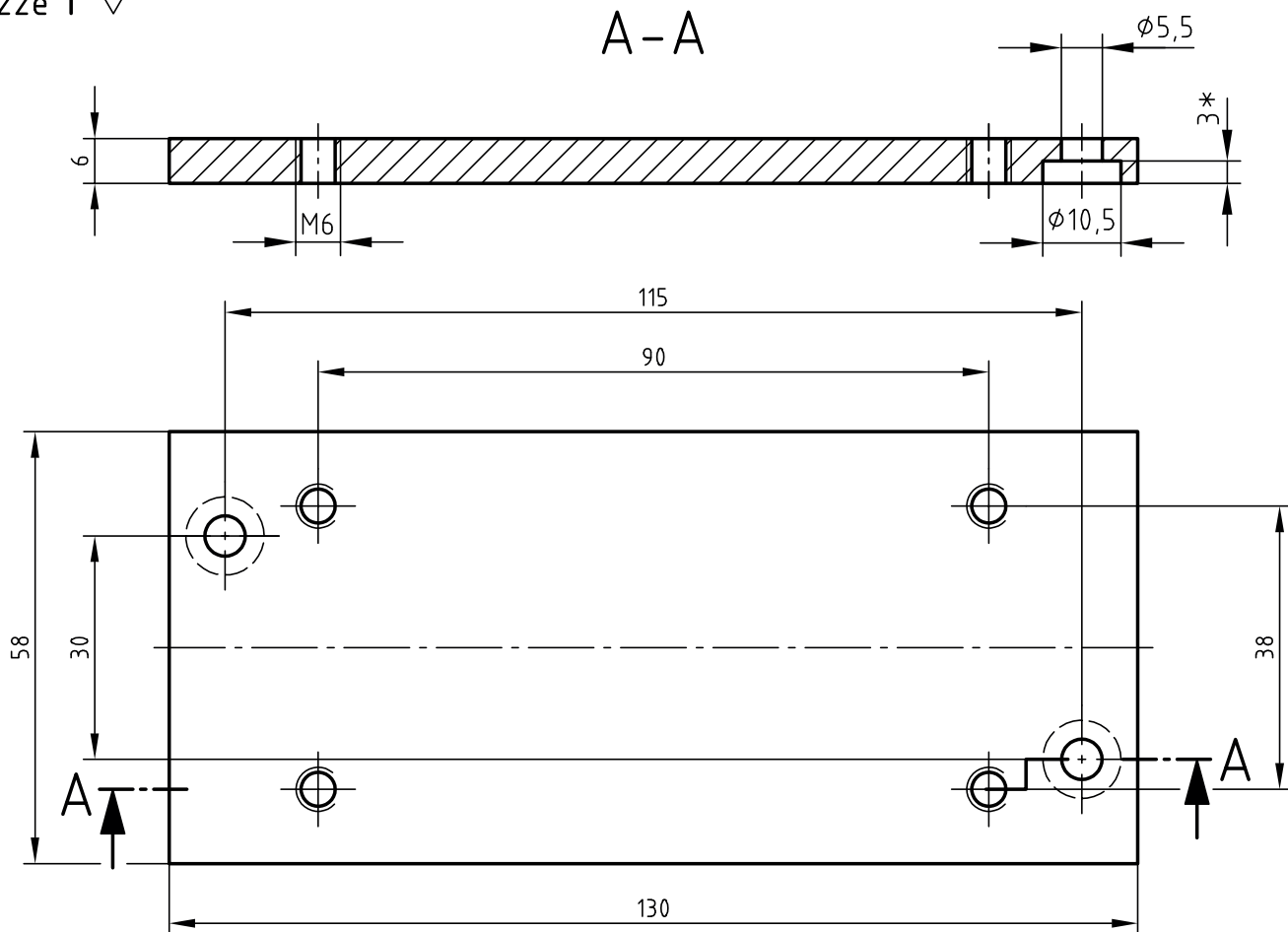
Skizze 1 \sqrt{Rz\ 16}
