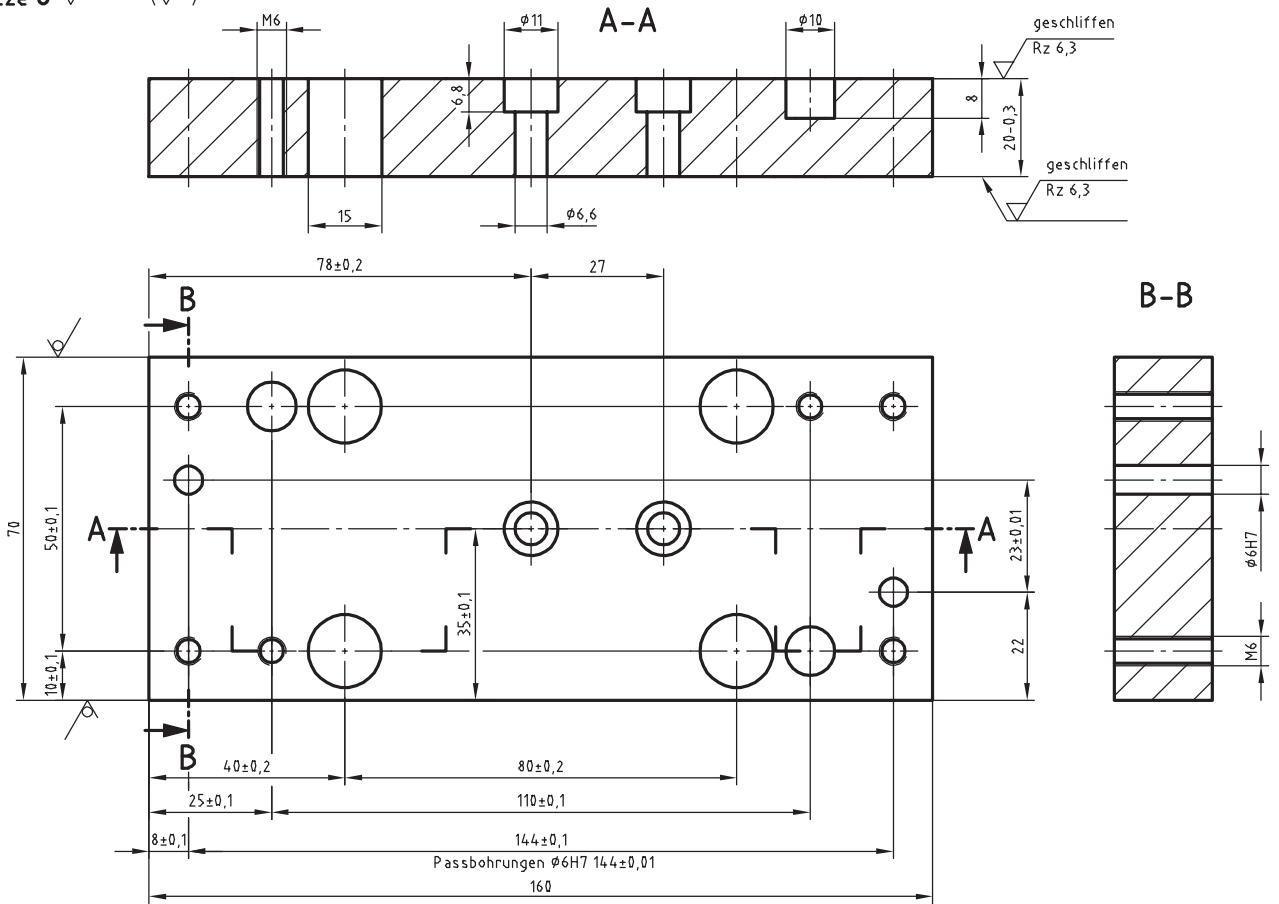
Skizze 8 \sqrt{Rz\ 16} ( \checkmark )
