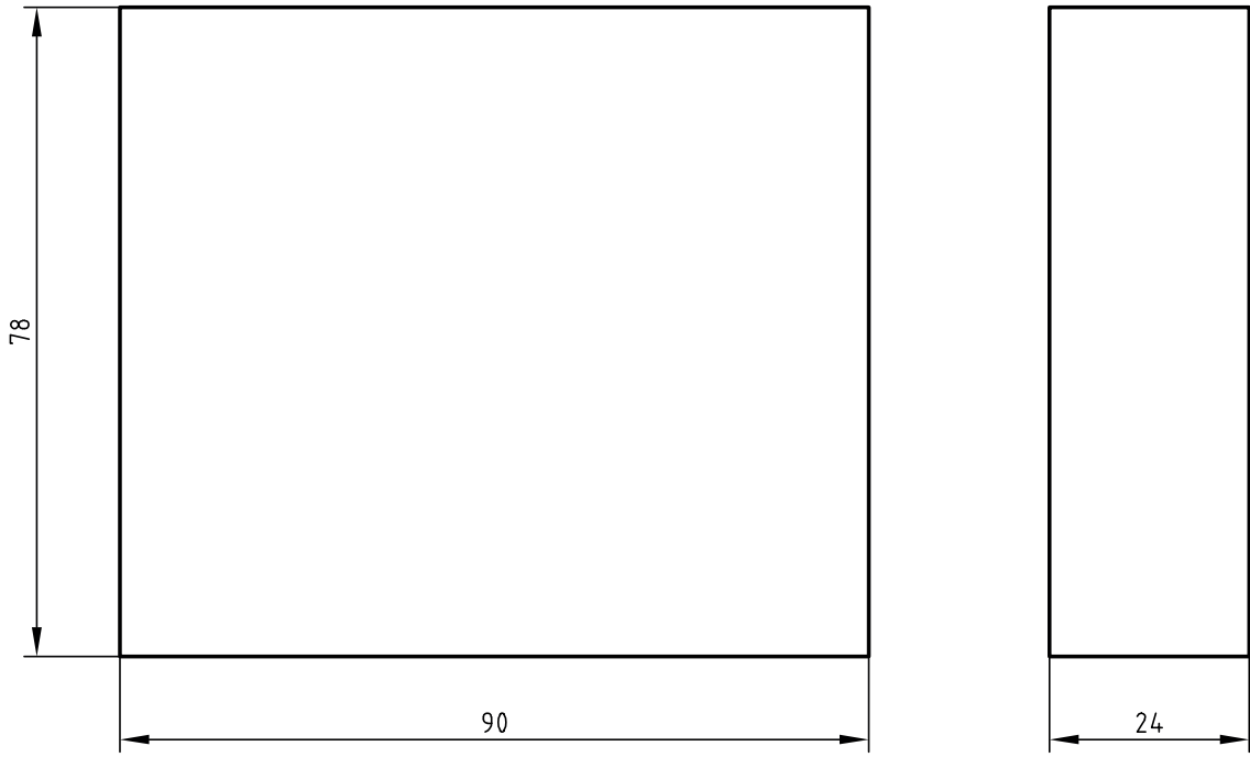
Skizze 1 \sqrt{\text{Rz 16}}
