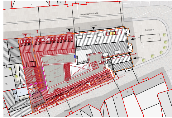
Lageplan mit Dachaufsicht
