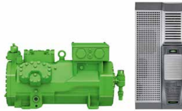
VARIPACK Frequenzumrichter eignen sich zur einfachen und sicheren Leistungsregelung
