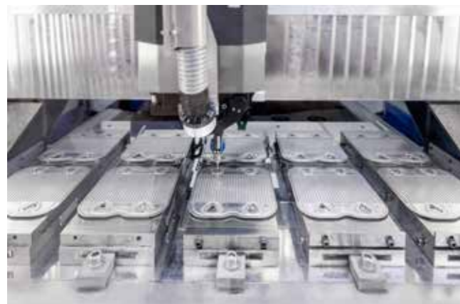
Produktion der Sunfire-Technologie
