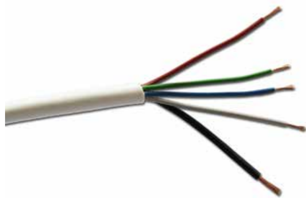
halogenfreies LED-RGBW-Kabel
