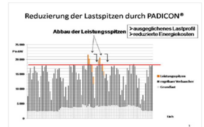
Mögliche Einsparung beim Leistungsbezug nach Optimierung
