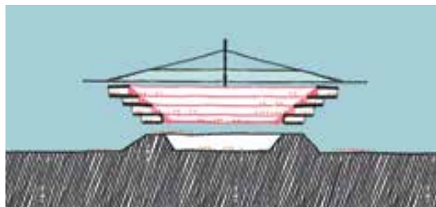
38. Das Olympiastadion als schematischer Querschnitt 2024
