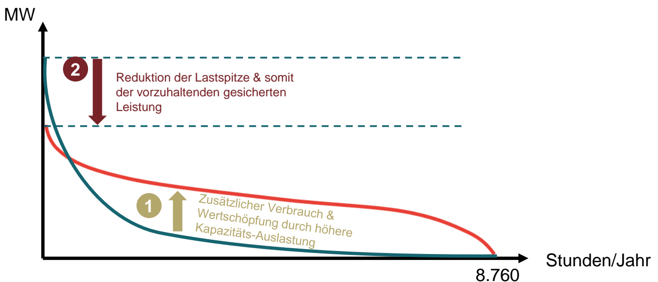
Abbildung 4. Vorteile einer Erschließung der Wertschöpfungs- und Flexibilitätpotenziale des Stromverbrauchs am Beispiel einer Lastdauerkurve (schematisch)
