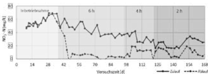
Abb. 2: Nitrat-N-Konzentration im Zulauf und Ablauf des Denitrifikationsreaktors bei unterschiedlichen Aufenthaltszeiten von 2-6 h im Denitrifikationsreaktor
